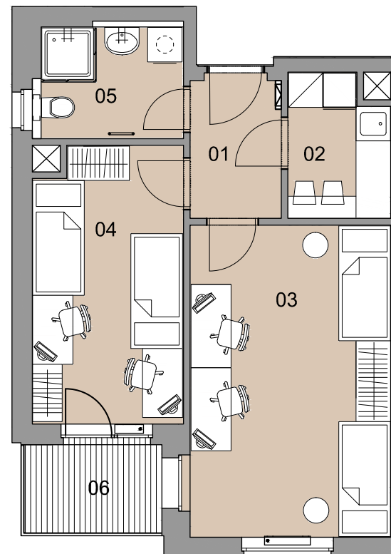
Typický byt 2+1
